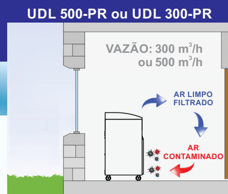
MODELO PISO RECIRCULAÇÃO DE AR
