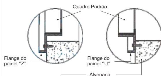
DETALHE DE FIXAÇÃO
