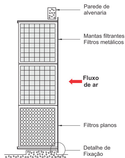
PERFIL
