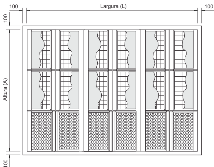
ELEVAÇÃO
