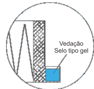
DETALHE A
