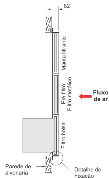
PERFIL
